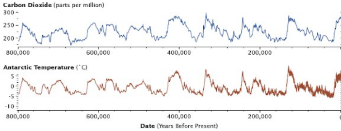
图 68 南极大气温度和大气二氧化碳含量变化图
