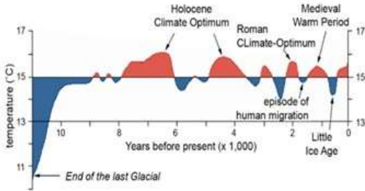
图 28 过去一万一千年大气温度变化图
