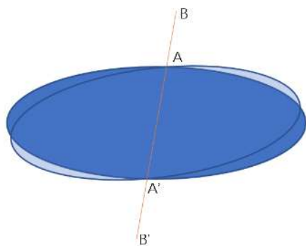
图 73 木星地球轨道盘相交示意图
