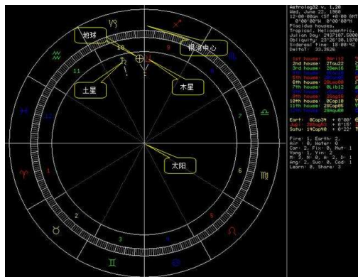
图 76 智利 9.5 级大地震时的星盘图
