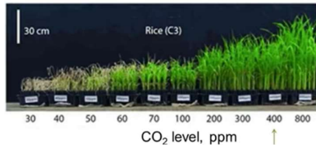
图 70 陆生植物生长状态和二氧化碳的关系图
