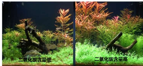
图 69 水生植物生长状态和二氧化碳的关系图
